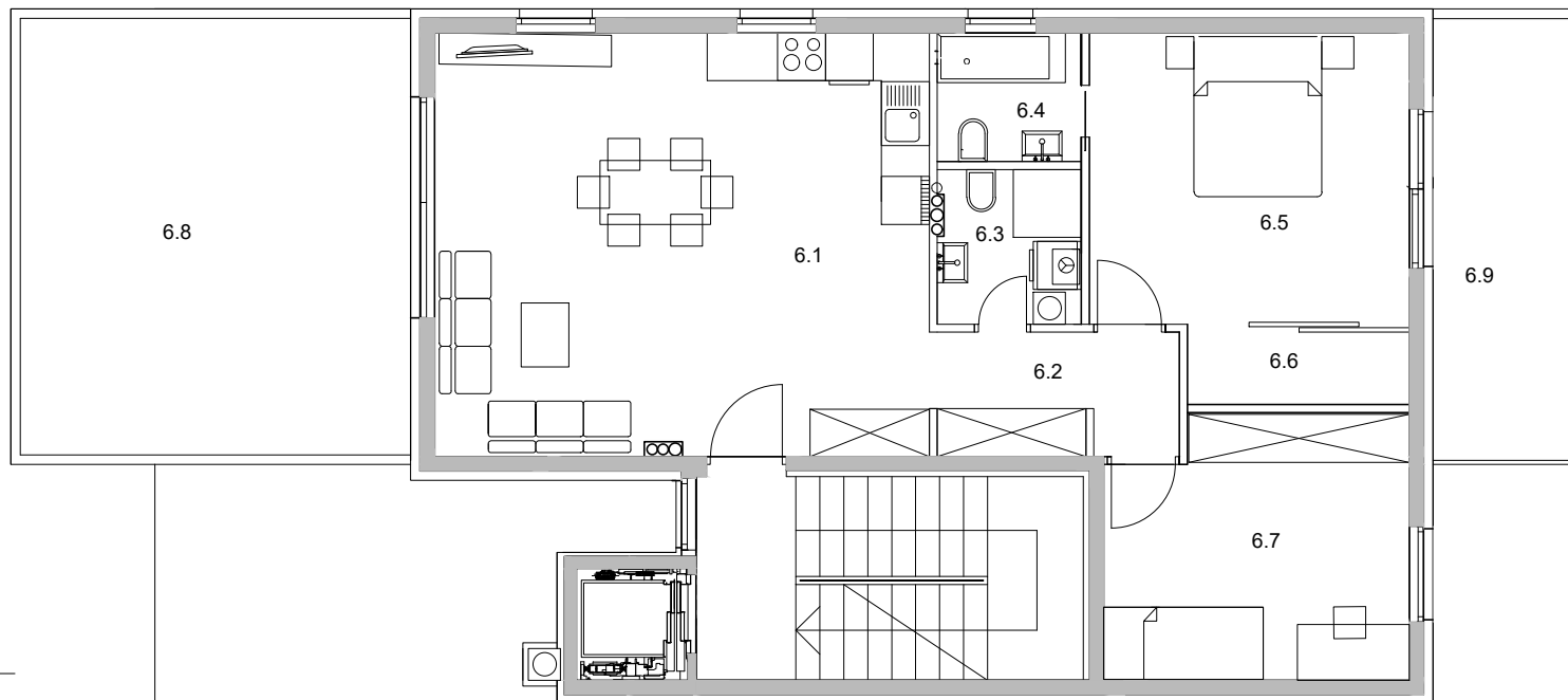
UVUČENI KAT
