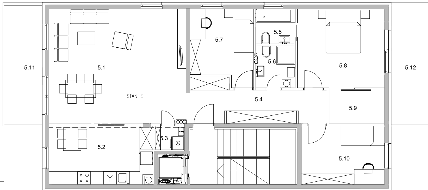
DRUGI KAT
